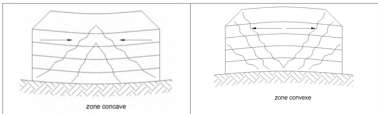
Illustration des effets de l'incurvation du sol sur le bâti
