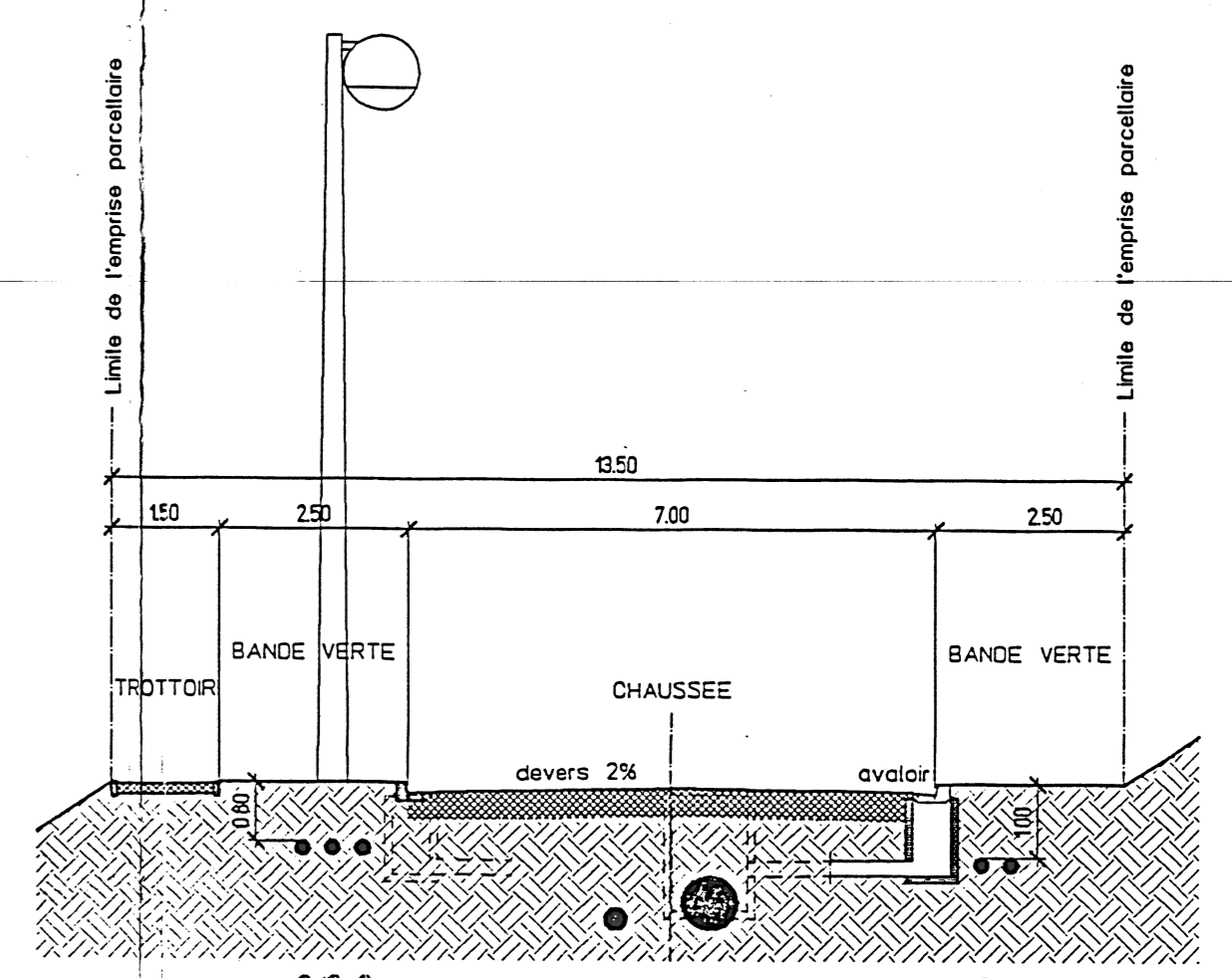
VOIRIES - UTILITES COUPE TYPE Ech. 1/100
