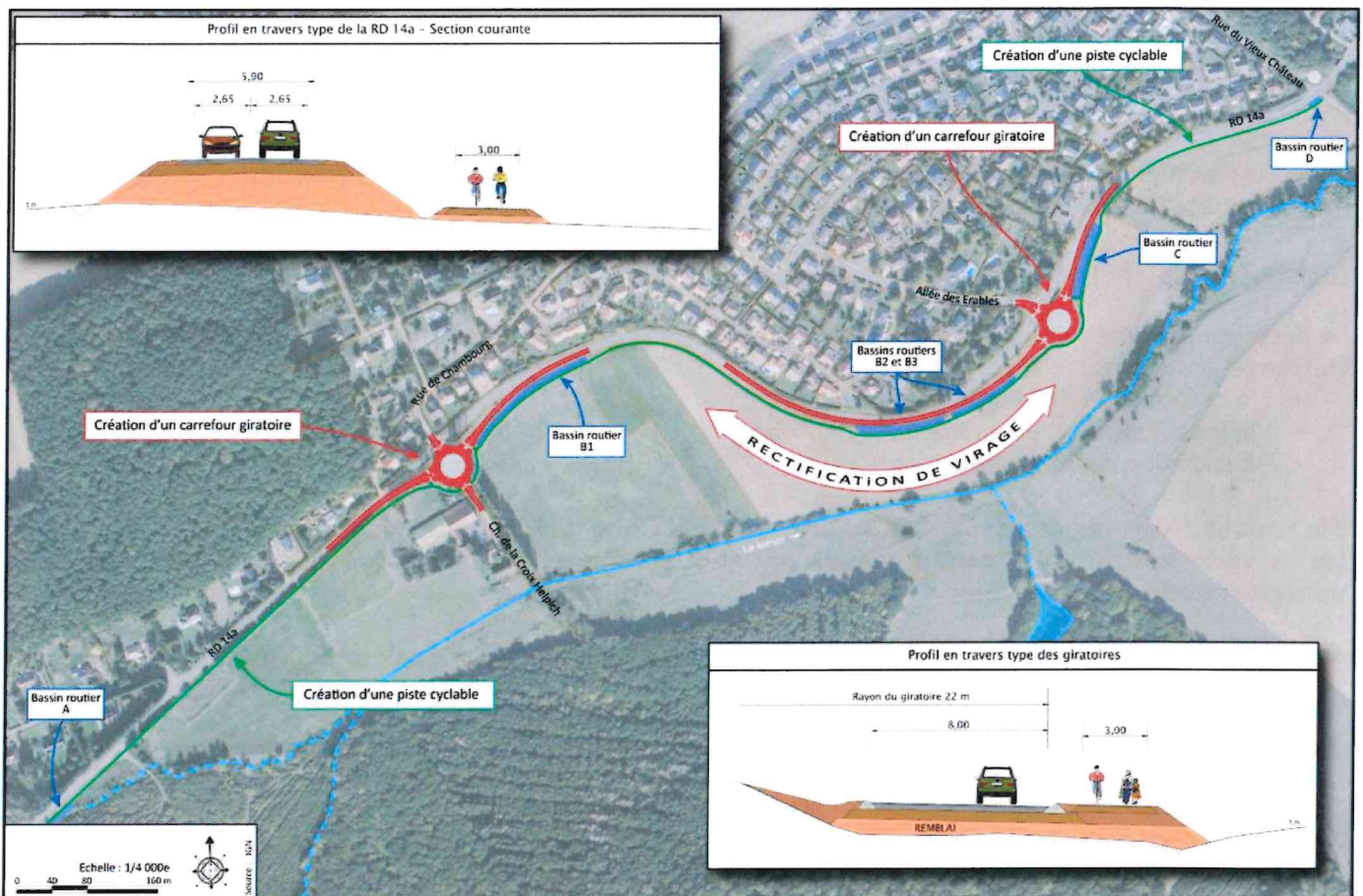
Figure 1: Plan général des travaux
