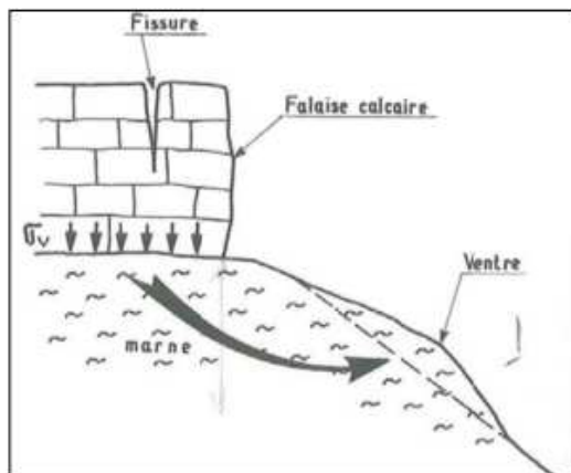
Illustration 4: Fluage d'après Philipponat & al. (Rapport BRGM)
