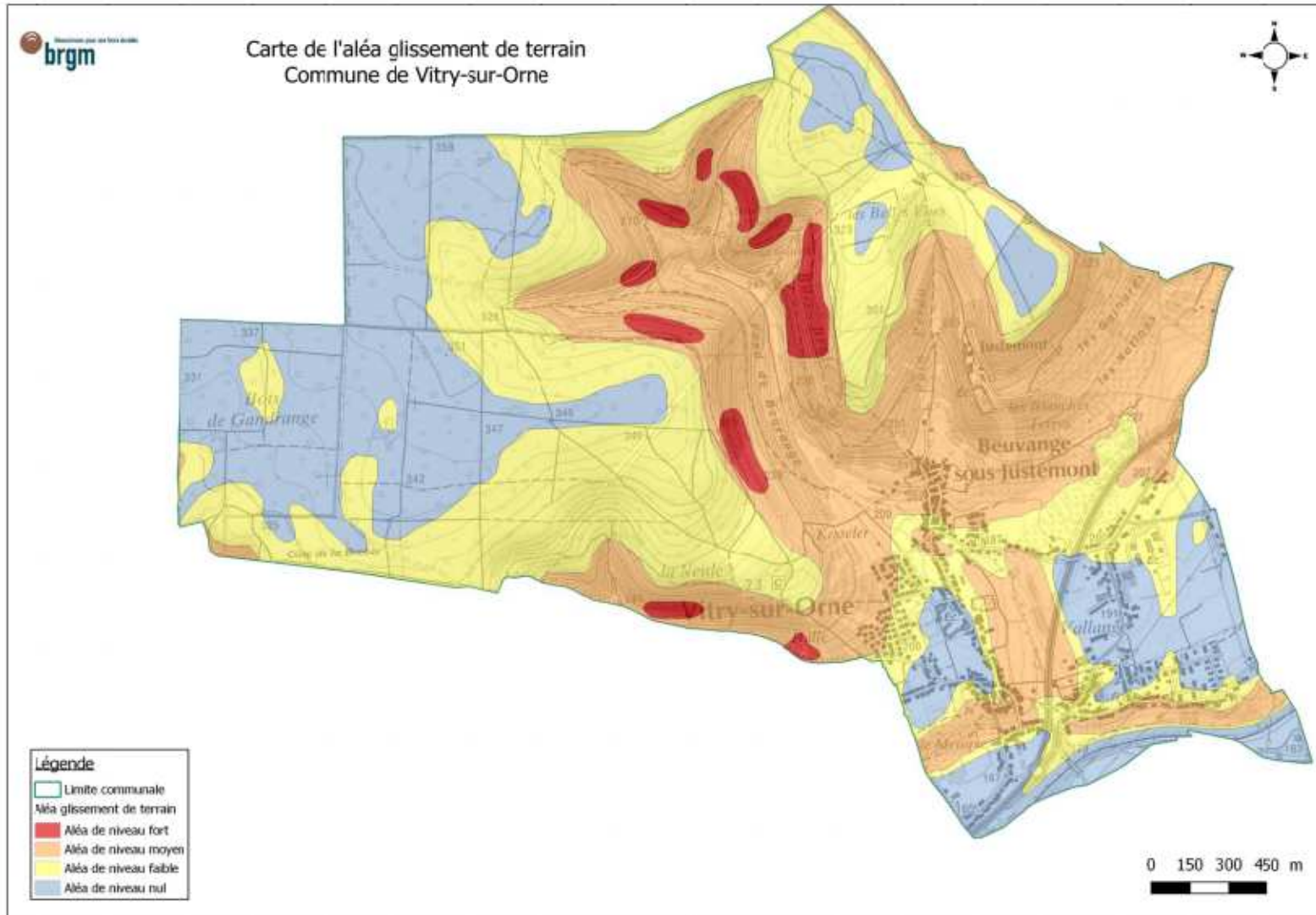
Illustration 8: Carte d'aléas sur Vitry-sur-Orne
