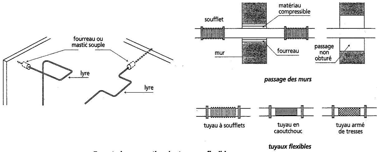
Tuyauterie : conception des tronçons flexibles.
