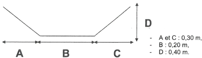
Extrait du dossier de déclaration - profil type du cours d'eau dévié
